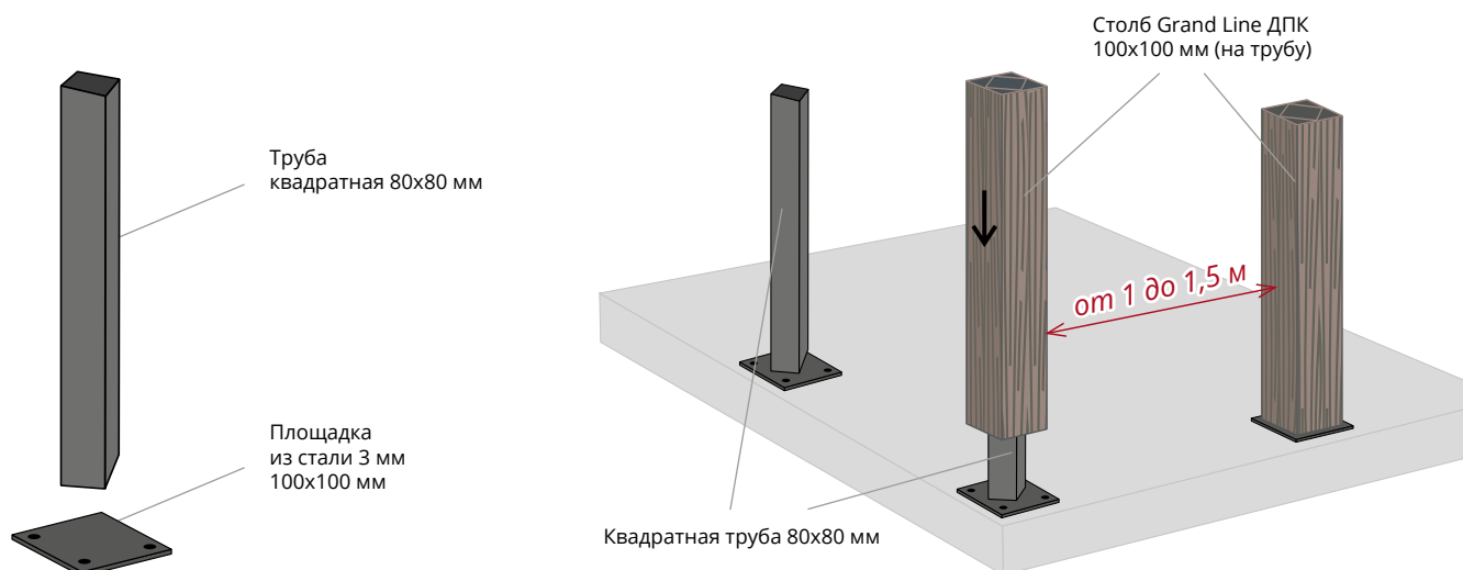
Пример изготовления армирующей площадки для столбов ДПК
