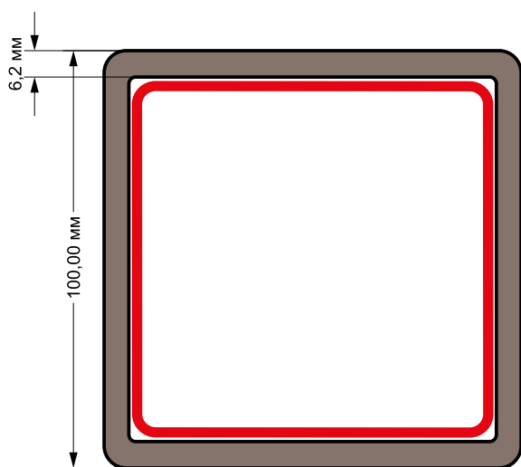
Установка столба ДПК на квадратную трубу 80x80 мм
